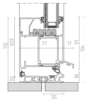
VLEUGEL GLAS (gesloten onderregel)
