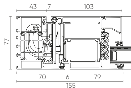
VLEUGEL GLAS ZIJ - verdoken scharnieren
