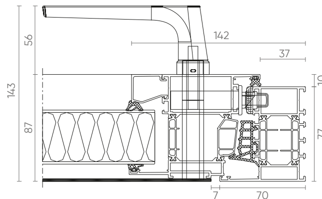
VLEUGEL PANEEL OVERDEKKEND KRIJK
