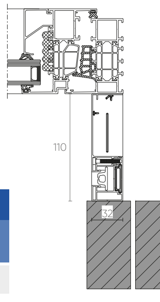
Montagemogelijkheden
