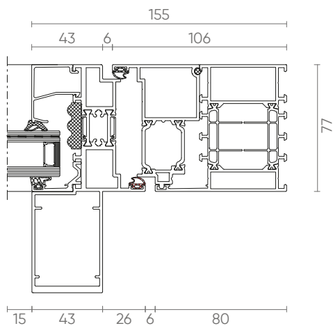
MASTERLINE PIVOT XL - ZIJ
