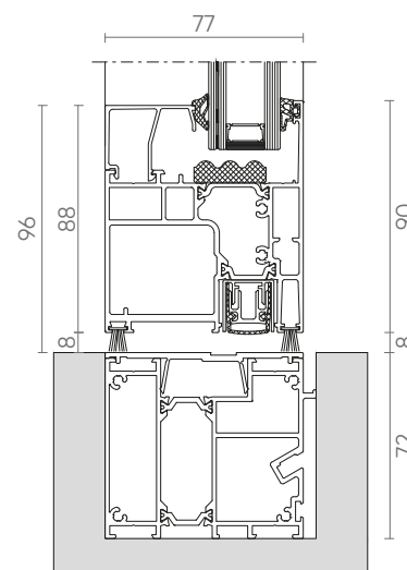
MASTERLINE PIVOT XL - ONDER
