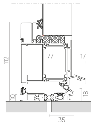
VLEUGEL PANEEL (gesloten onderregel)
