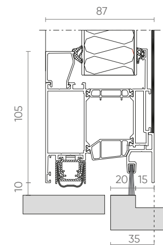
VLEUGEL PANEEL OVERDEKKEND ONDER
