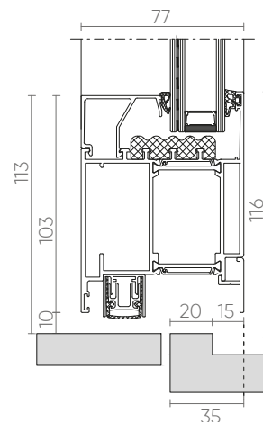
VLEUGEL GLAS (automatische tochtborstel)
