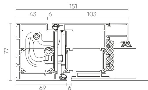
VLEUGEL PANEEL ZIJ - verdoken scharnieren
