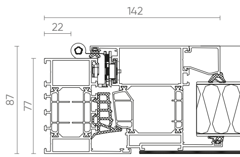
VLEUGEL PANEEL OVERDEKKEND ZIJ
