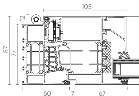
VLEUGEL GLAS ZIJ - inlegscharnieren
