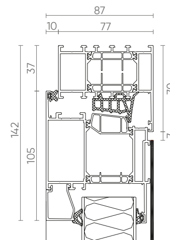
VLEUGEL PANEEL OVERDEKKEND BOVEN
