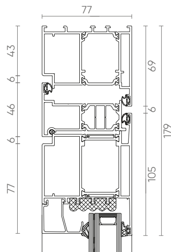
MASTERLINE PIVOT - BOVEN
