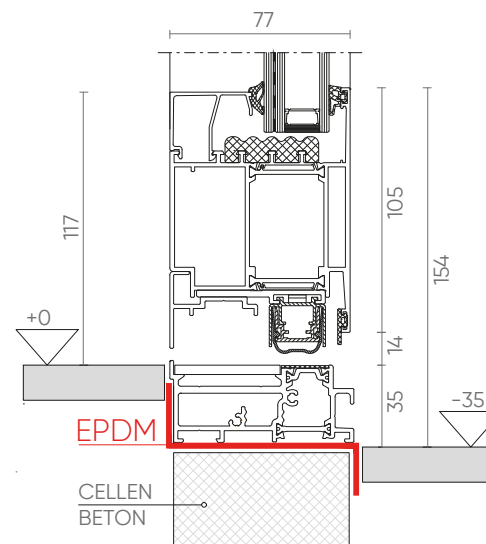
MASTERLINE PIVOT - ONDER
