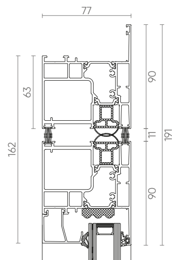
MASTERLINE PIVOT XL - BOVEN
