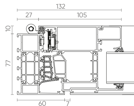
VLEUGEL PANEEL ZIJ - inlegscharnieren
