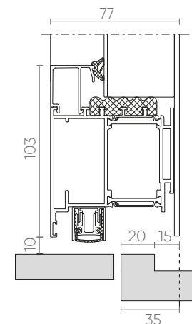
VLEUGEL PANEEL (automatische tochtborstel)
