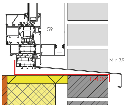
RAAMDORPEL + ROLLUIGGELEIDER
